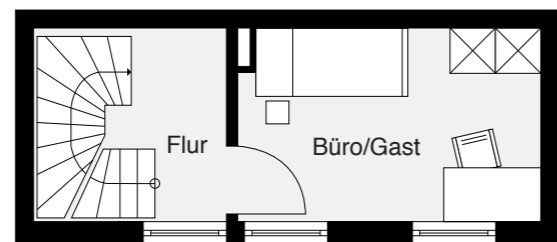
ERDGESCHOSS
